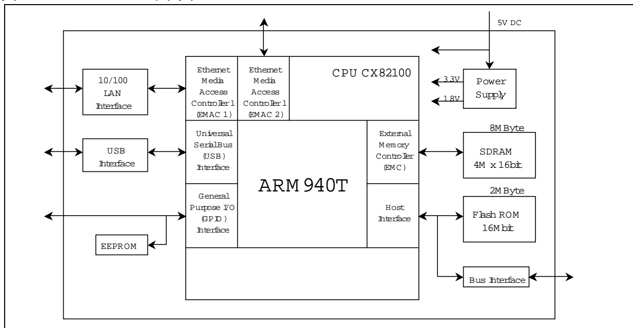
図1. JAMP-STD ブロック図
