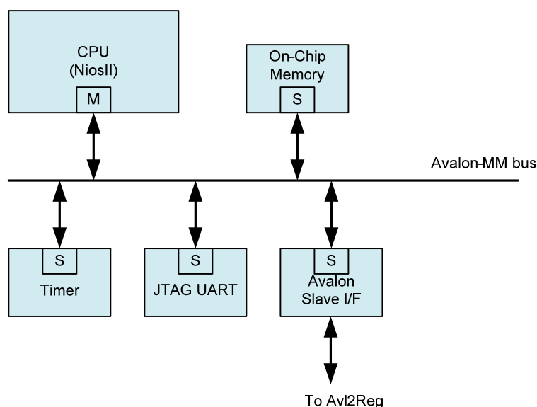
図 2: リファレンス・デザインの CPU システム
