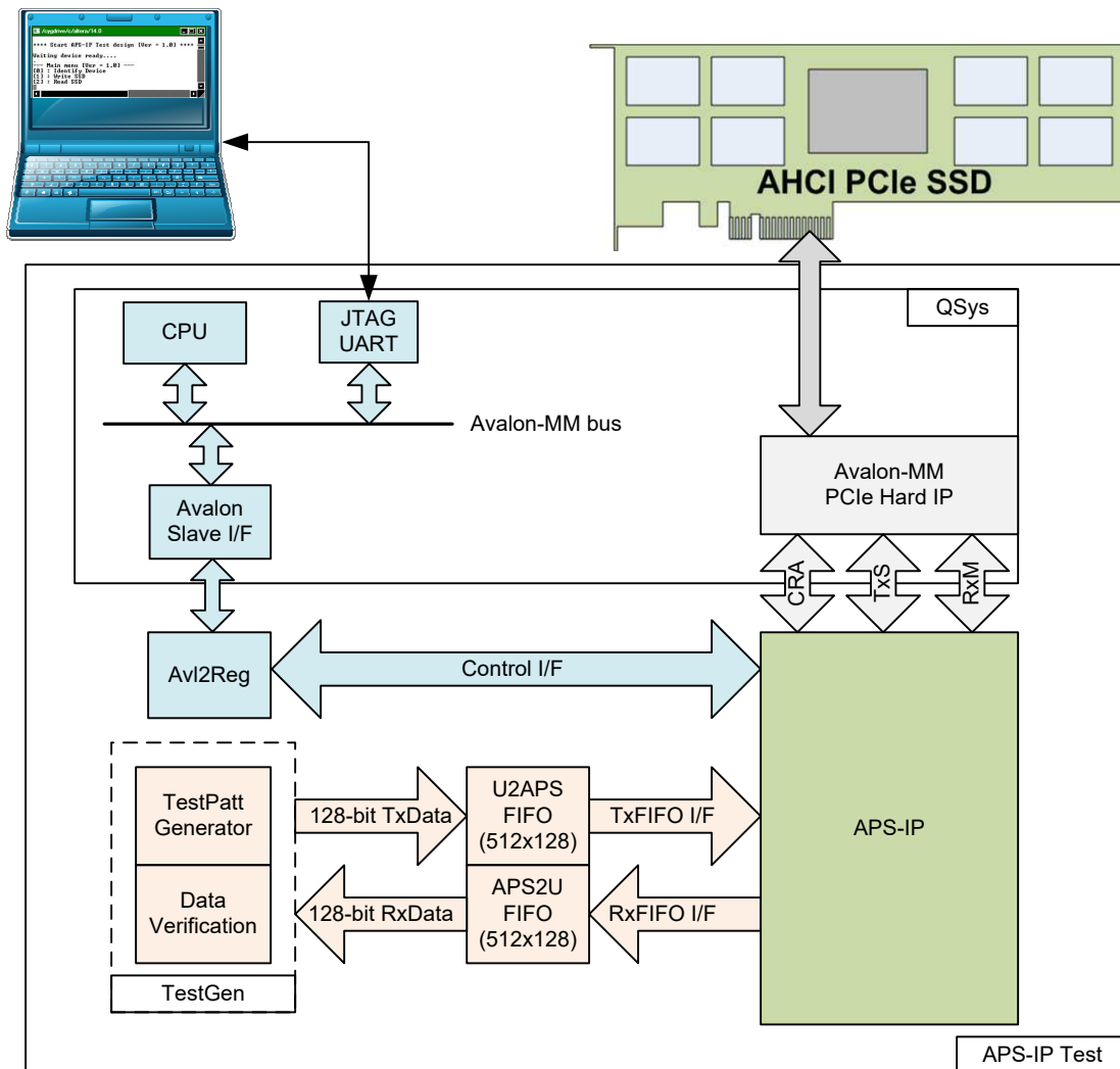
図 1: APS-IP リファレンス・デザインのブロック図
