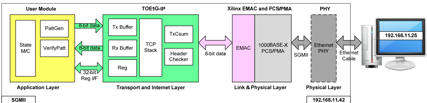
図 3 SGMII (VC707/Zynq Mini-ITX)のハードウェア構造
