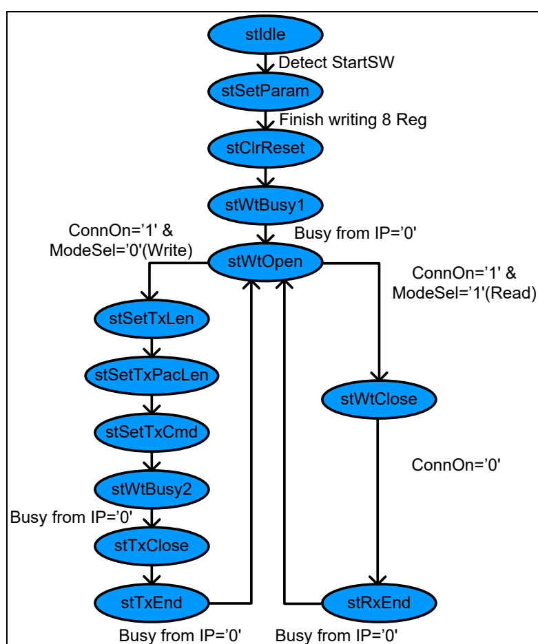
図 5: ユーザ回路内ステートマシンの状態遷移図
