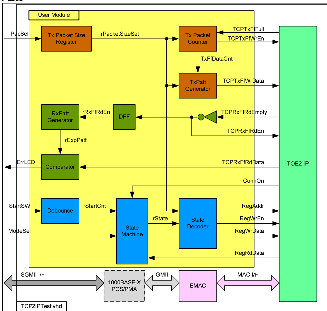
図 4: リファレンス・デザインの利用者回路ブロック図
