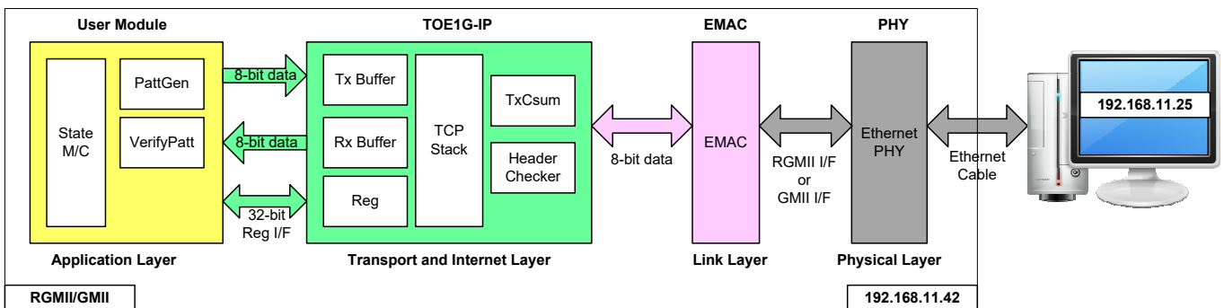
図 2: RGMII または GMII (AC701/KC705)のハードウェア構造
