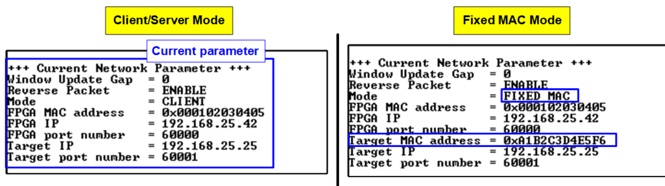
Figure 3-2 Display current parameter result
