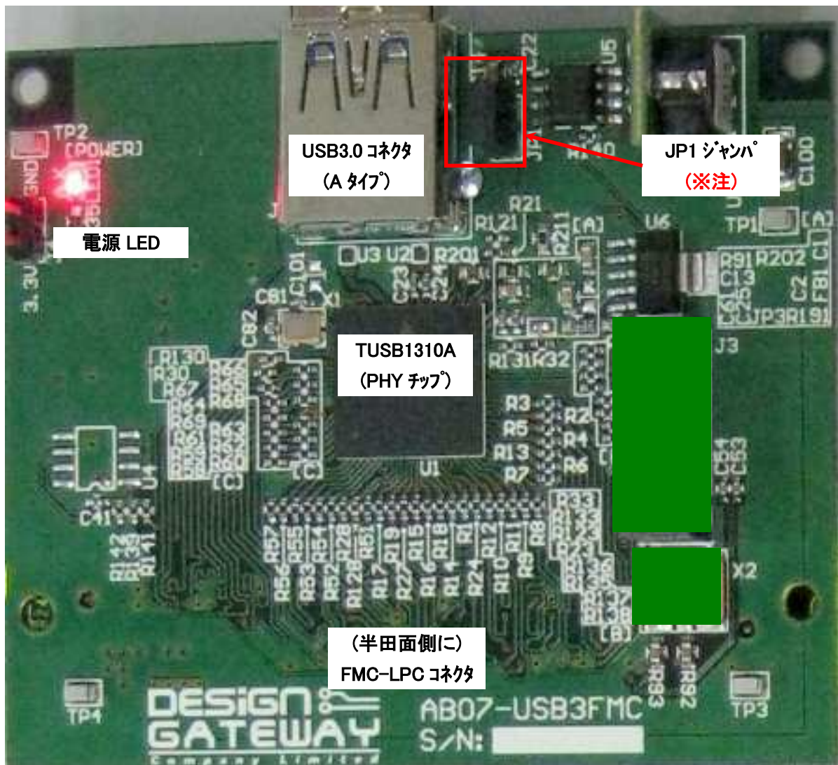
図 1: AB07-USB3FMC/AB07-USB3FMC-1.8VIF 基板の外観
