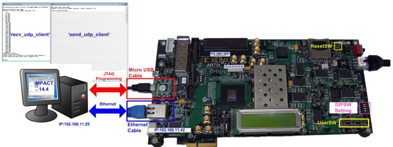
図 1: AC701 ボードでの UDP1G-IP デモ環境
