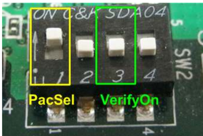
図 2-1: 本デモにおけるディップ・スイッチ
