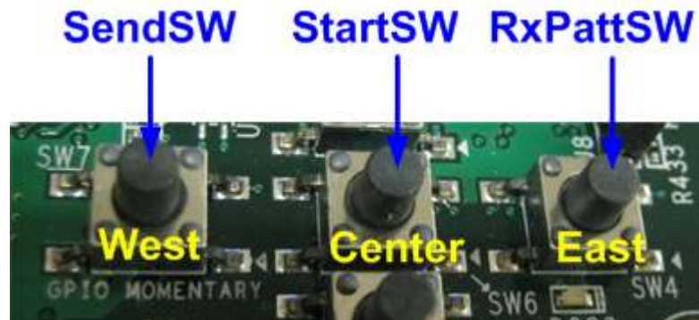
図 2-3: 本デモで使用する押しボタン
