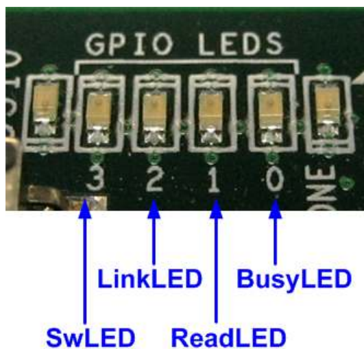
図 2-2: 本デモにおけるLED
